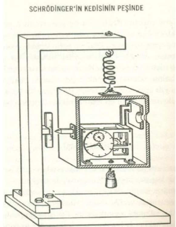
Şekil 9.1 "Kutudaki saat" deneyi. Deneyi pratikte uygulayabilmek için gerekli ıvır zıvır (ağırlıklar, yaylar vs.) enerjisiyle zamanın birlikte ölçümündeki belirsizliği kaldırmayı daima imkânsız kılar.
